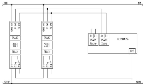
Rys Nr 16 Przykład dla układu pojedynczy nawiew, pojedynczy wywiew
