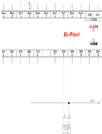
Rys Nr 3 Podłączenie sygnału z dodatkowego presostatu filtra dokładnego (styk normalnie otwarty (NO))
