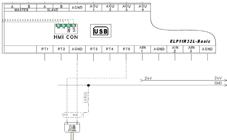
Rys. Nr 13 Podłączenie czujnika temperatury powrotu wody (montowany na kolektorze wymiennika) do sterownika
