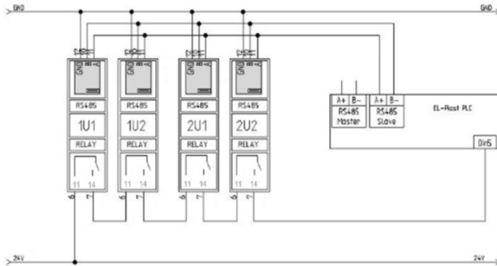
Rys Nr 19 Przykład dla układu podwójny nawiew, podwójny wywiew
