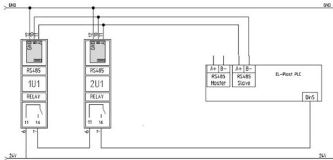
Rys Nr 20 Przykład dla układu pojedynczy nawiew, pojedynczy wywiew
