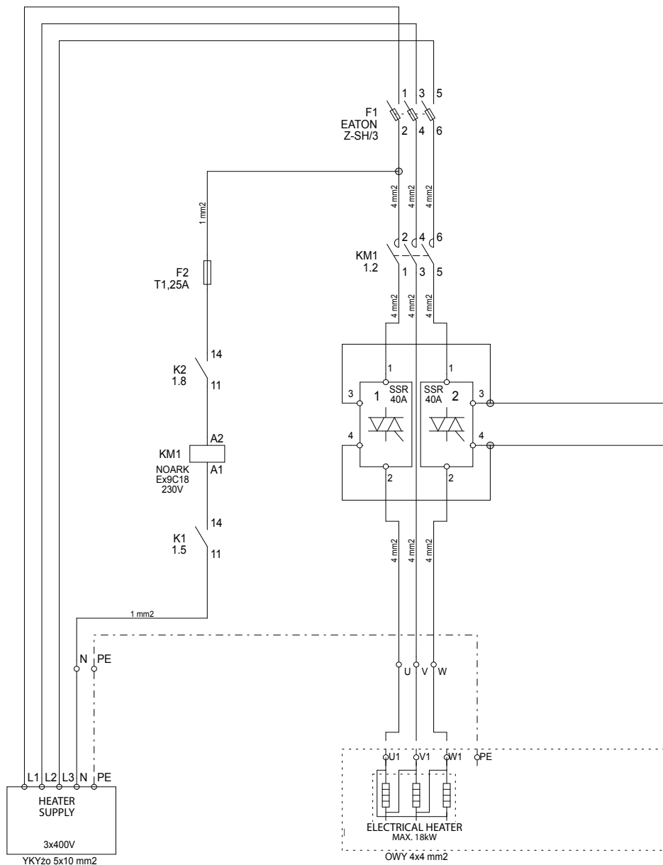
Fig. No 25 Module EH-M-18kW/1
