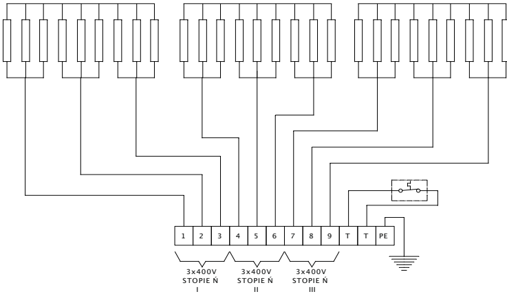
Rys Nr 29 Schemat podłączenia grzałek w nagrzewnicy 324-3
