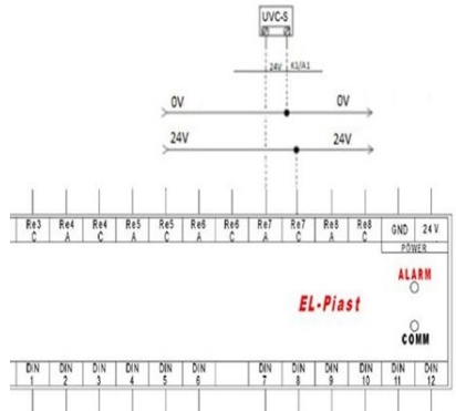
Rys Nr 5 Podłączenie sterowania lamp UV-C
