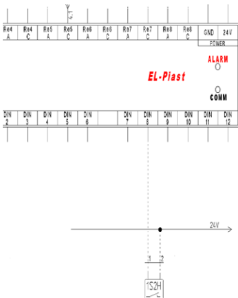
Рис. № 3 Подключение сигнала от дополнительного точного контроля давления фильтра (обычно открытый контакт (NO))
