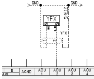
Rys. Nr 10 Podłączenie sygnału sterującego do sterownika
