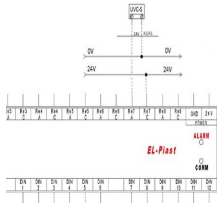
Рис. №5 Подключение управления UVC-S лампами
