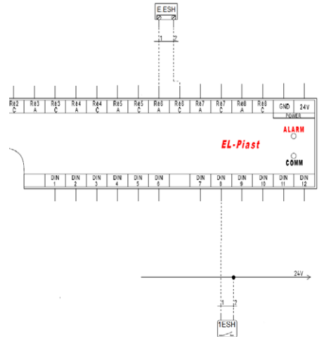
Рис. № 4 Контроль работы электростатического фильтра
