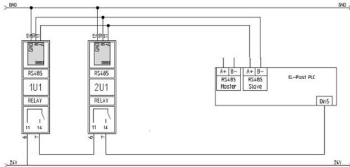
Рис. № 20 Пример для системы с одиночной подачей и одиночной вытяжкой воздуха
