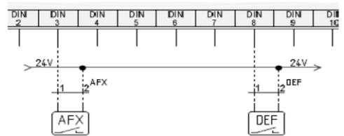
Рис. № 12 Подключение к контроллеру сигнала возврата сигнала тревоги и размораживать
