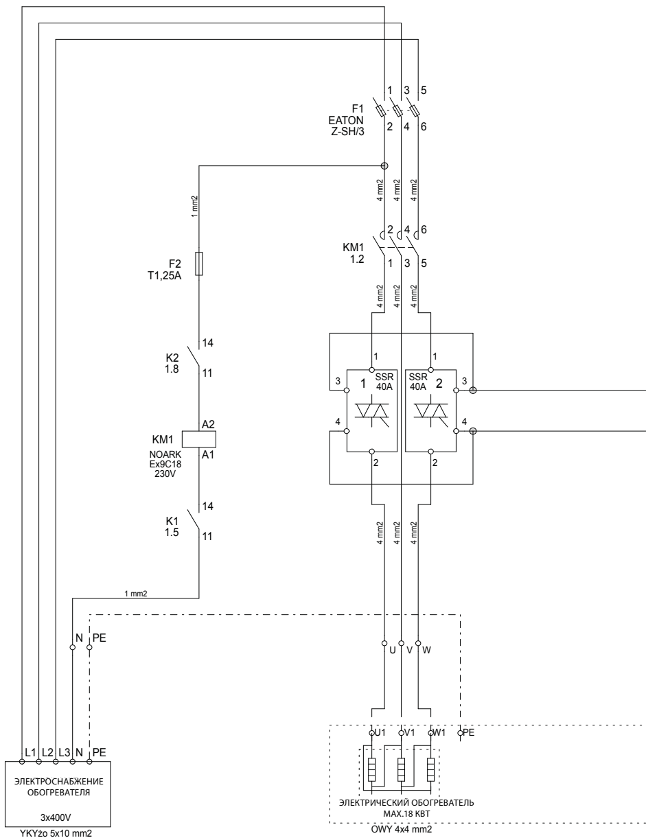
Рис. № 25 Модуль EH EVO-T 18 кВт
