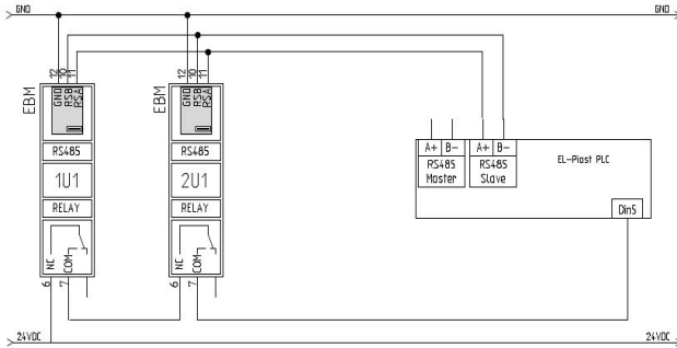
Rys Nr 18 Przykład dla układu pojedynczy nawiew, pojedynczy wywiew
