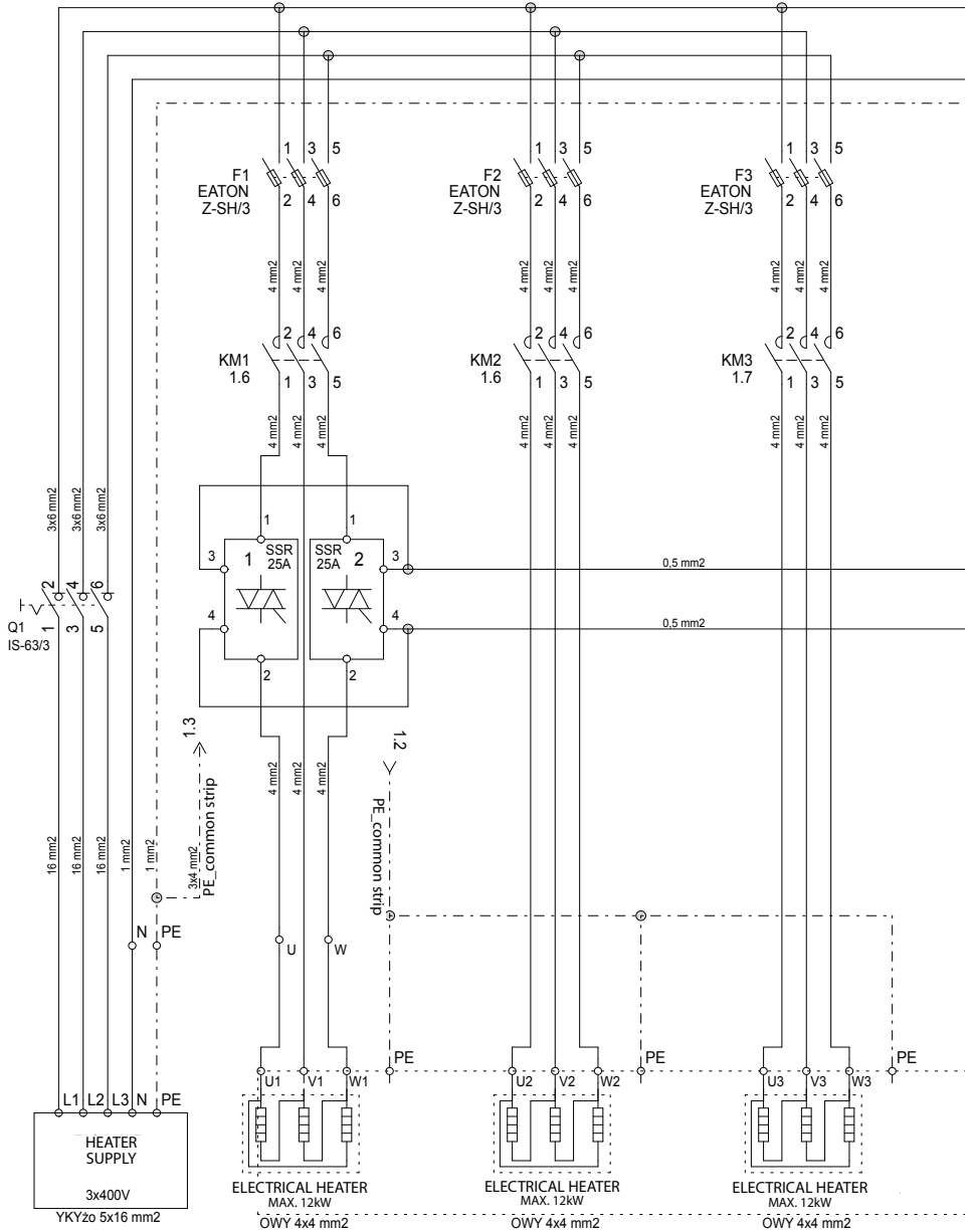
Fig. 26 Module EH-M-36 kW/3
