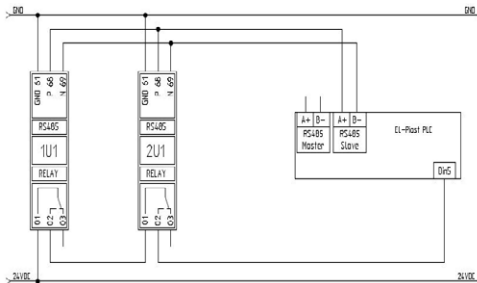
Рис. № 16 Пример для системы с одиночной подачей воздуха, одиночным выпуском воздуха
