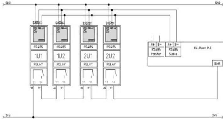
Рис. № 19 Пример для системы с двойной подачей и двойной вытяжкой воздуха
