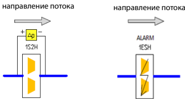
Рис. № 2 Дополнительное давление на точный фильтр или сигнальный контакт электростатического фильтра
