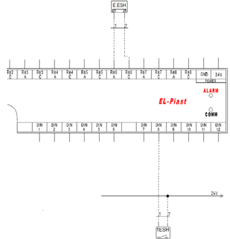
Rys Nr 4 Kontrola zabrudzenia filtra dokładnego lub kontrola pracy filtra elektrostatycznego
