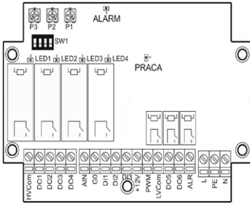
Rys. Nr.36 Moduł sterujący nagrzewnicą elektryczną HE
