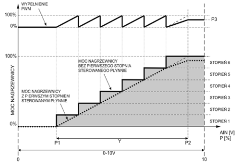
Rys. Nr. 39 Przebieg regulacji grzania
