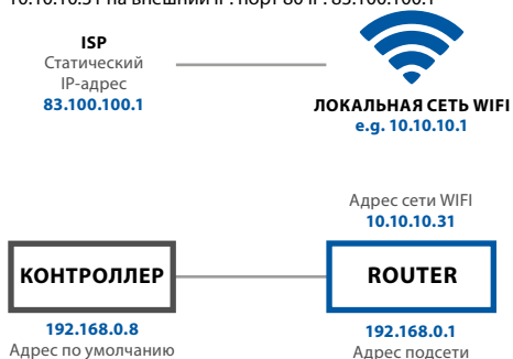
Рис. 17 Подключение контроллера через локальную сеть WiFi с внешним общим доступом
