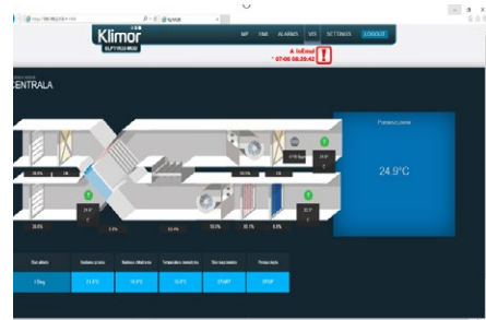
Rys. Nr. 13 Ekran wizualizacji centrali (w sterownikach ELP11R3ZL+)
